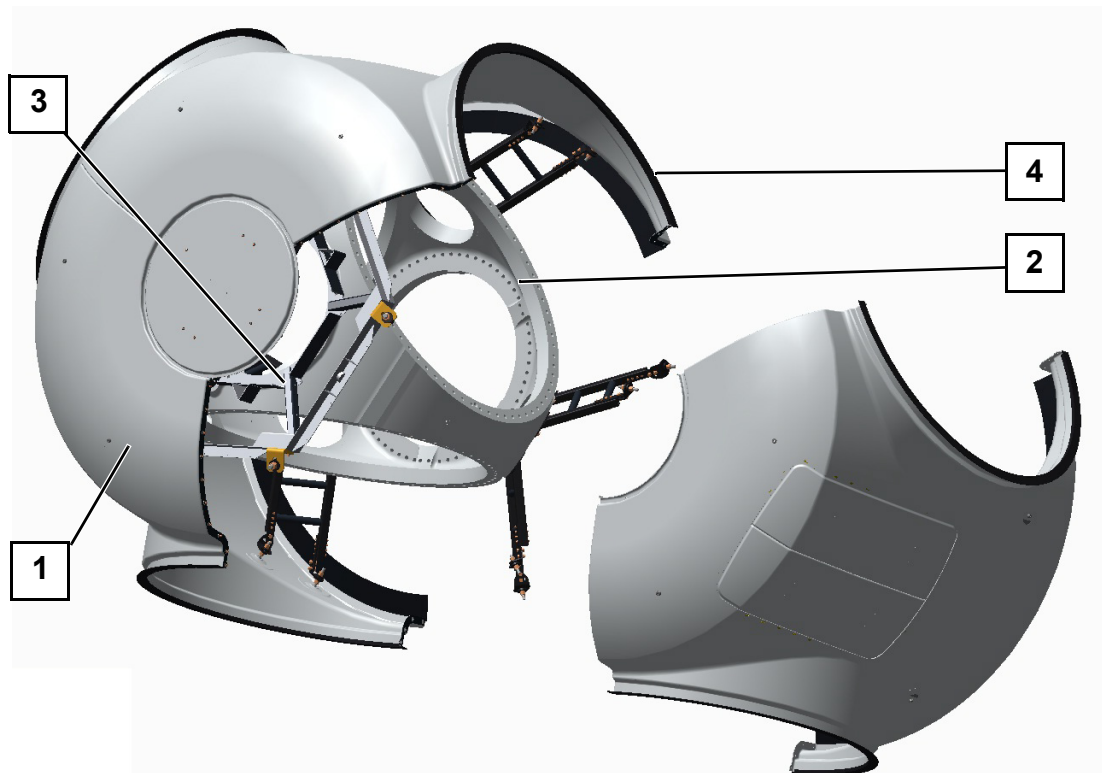
Abb. 2 Nabe und Spinner der Nordex Anlagen der Delta-Generation
