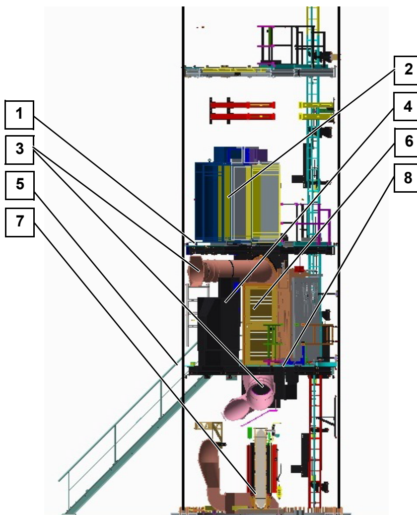
Abb. 1 Schnitt durch den Turmfuß, Variante Trafo im Turm
