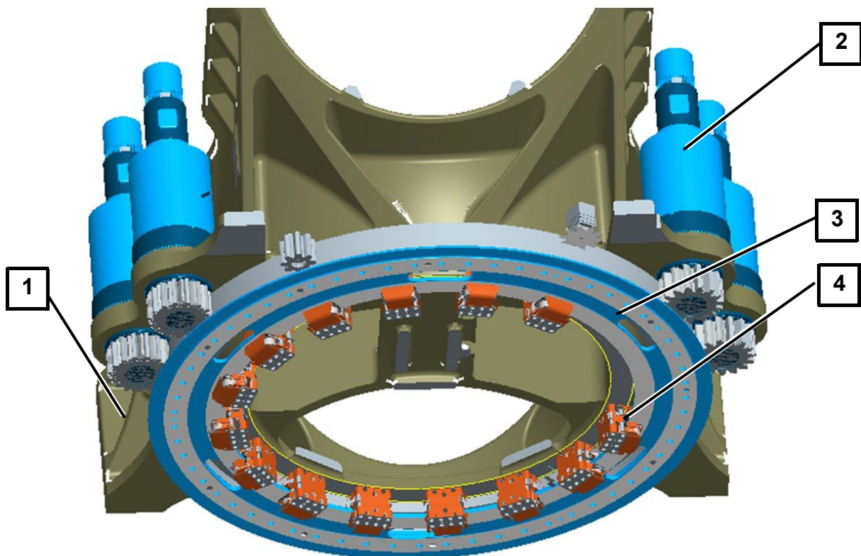
Abb. 4 Komponenten des Azimutsystems
