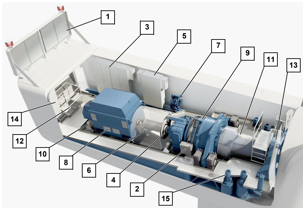
Abb. 3 Übersichtszeichnung Maschinenhaus
